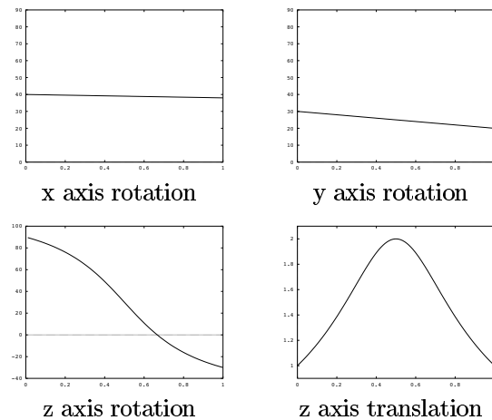
Fig. 15. Robot trajectories for linear case
